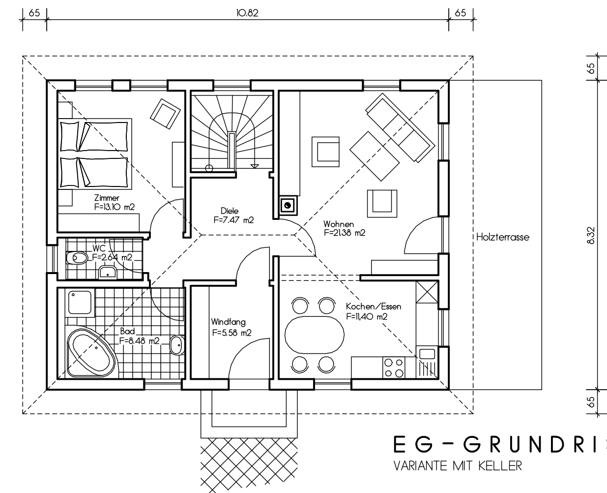
EG - GRUNDRISS VARIANTE MIT BODENPLATTE
